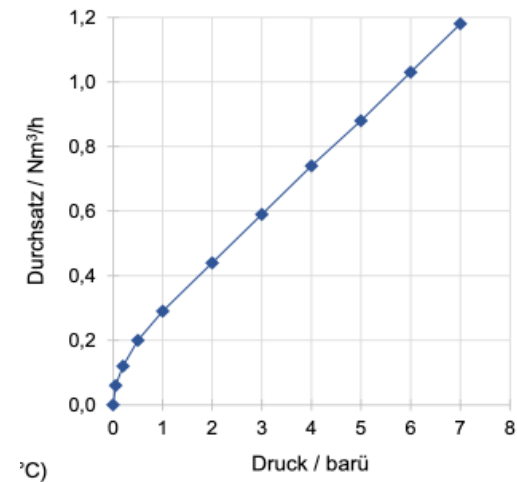
Strömungsmessungen bei Abströmen in die Umgebung Versuchsaufbau nach DIN EN 60534-2-3
